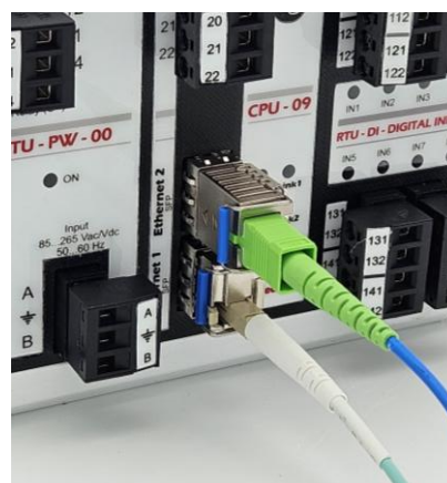
Figura 48 – 1 Fibra Bidirecional conexão SC + 1 Fibra Bidirecional conexão LC - PA1170B + PA1171B
