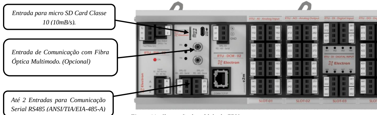
Figura 11 - Ilustração do módulo de CPU
