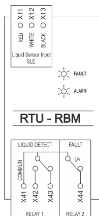
Figura 30 – Diagrama de Ligação - RBM
