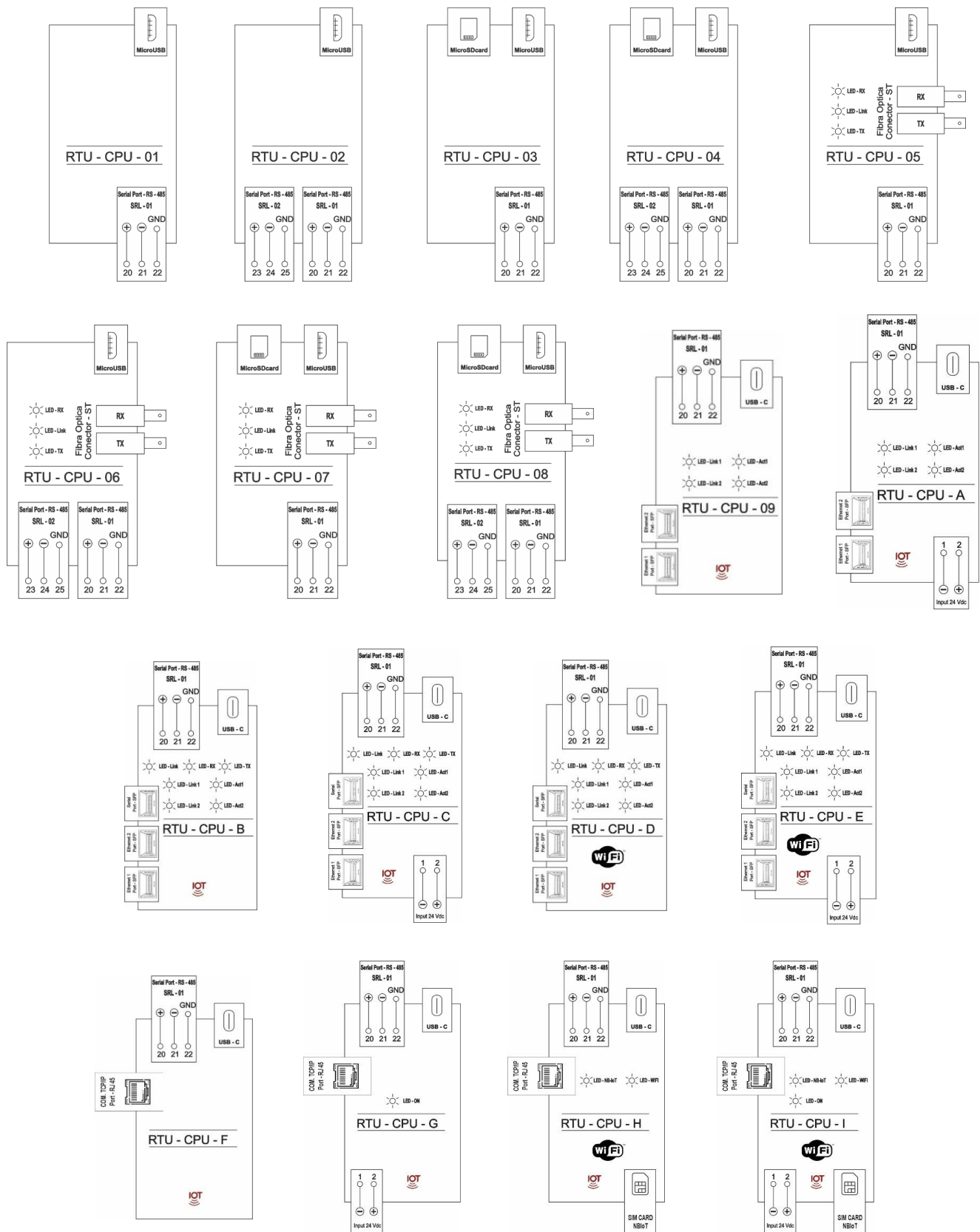
Figura 12 – Módulos CPU
