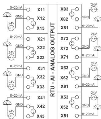
Figura 22 - Diagrama de Saída - Passiva
