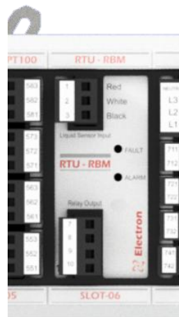
Figura 31 – Ilustração Módulo - RBM
