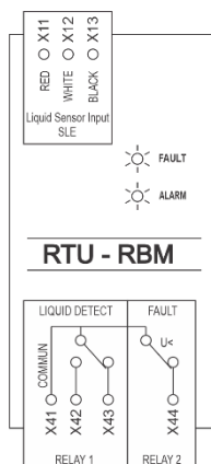
Figura 30 – Diagrama de Ligação - RBM
