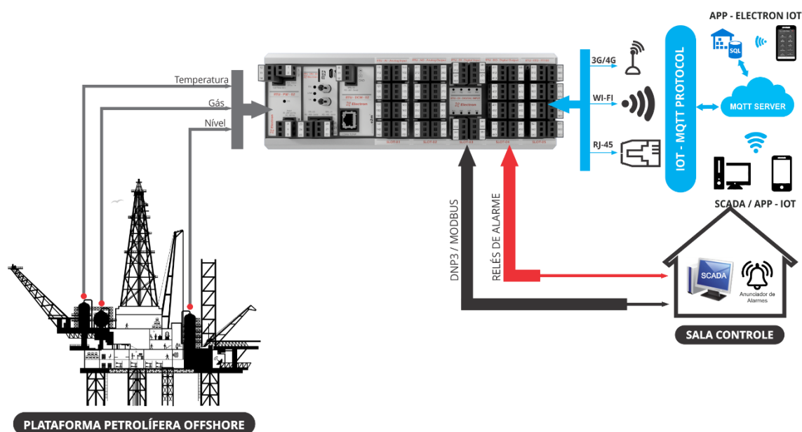
Figura 2 - Monitoramento e Proteção em Plataformas Petrolíferas Off-Shore
