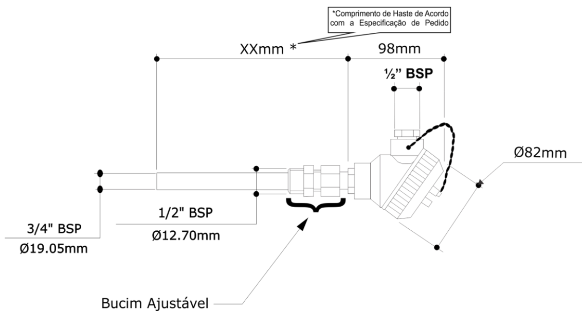
Imagem 2 – Dimensão Cabeçote
