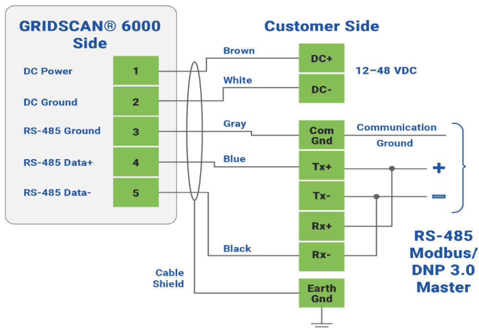
Fig 3 – Diagrama de conexão
